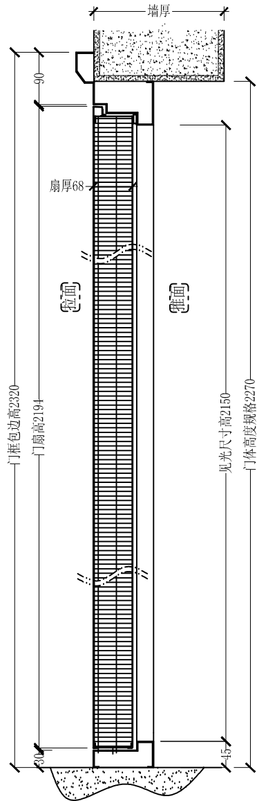
竖剖示意图
