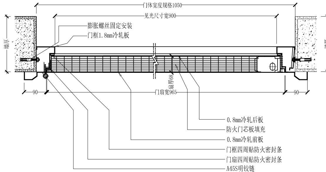
横剖示意图
