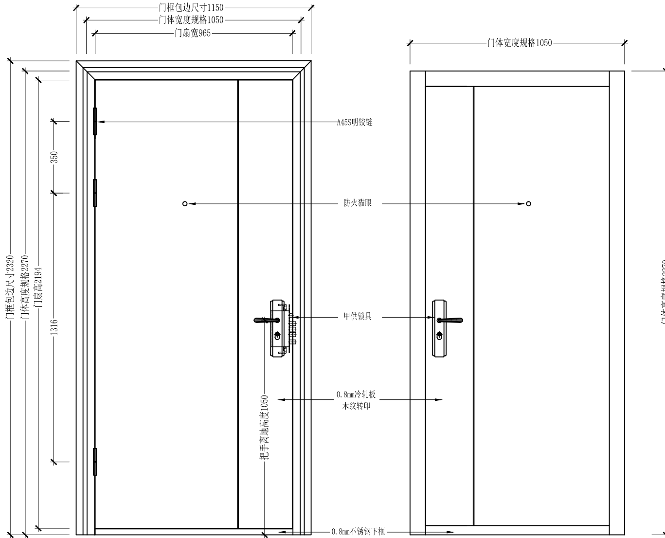
进户门推面立面示意图
